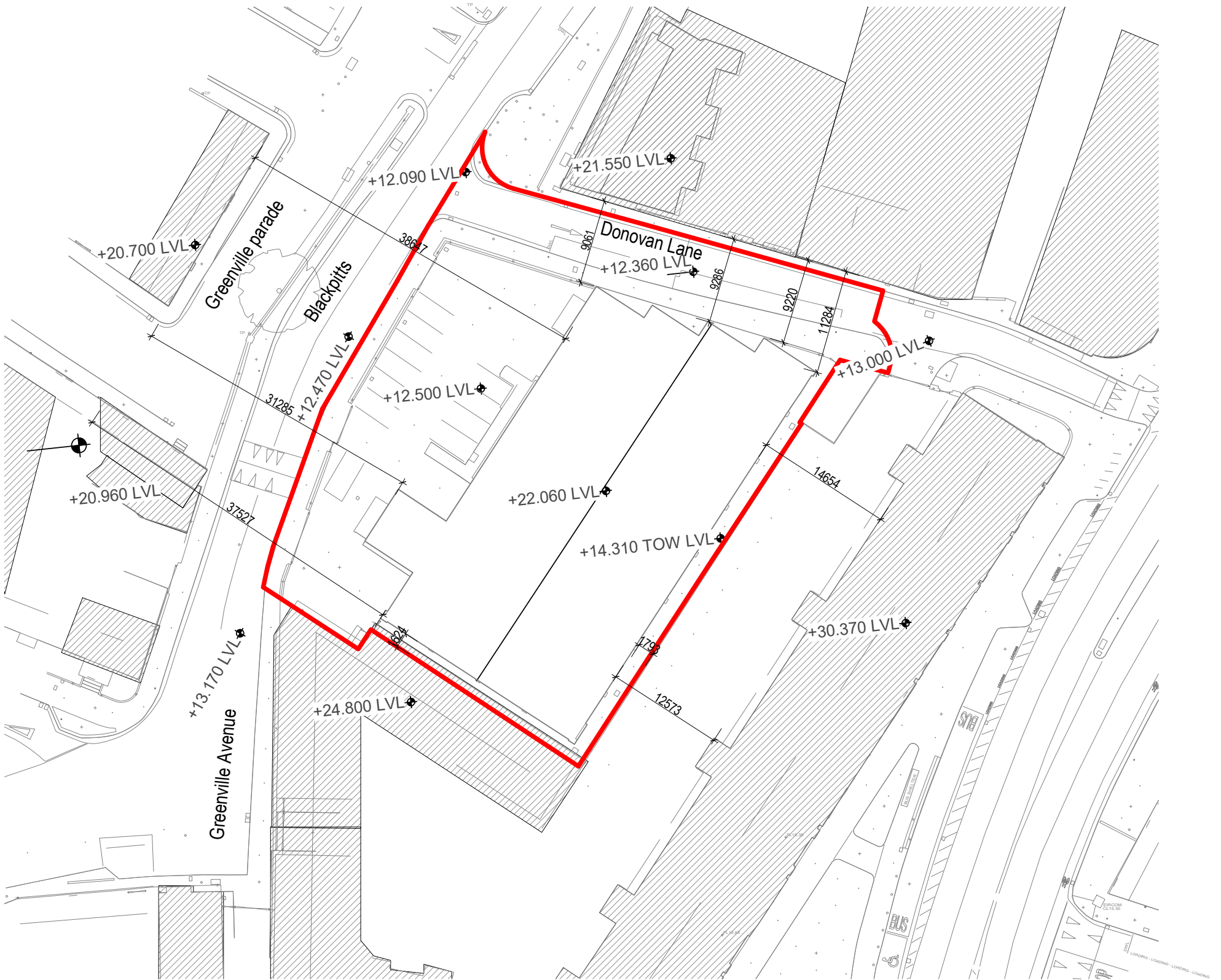
1 Existing Site Layout Plan Scale 1 : 500
